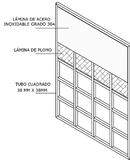
ARMADO - VISTA ISOMÉTRICA ESC. 1.25
