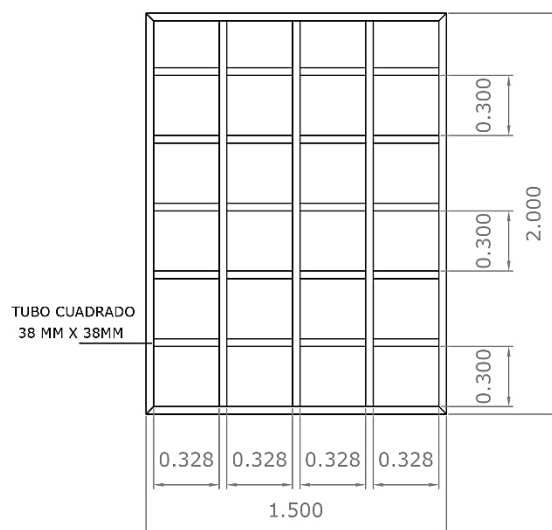
ESTRUCTURA - VISTA FRONTAL ESC. 1.25
